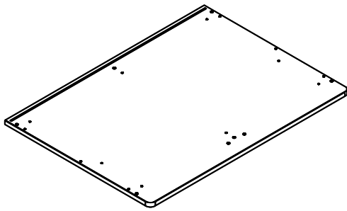
1 Top x1 (79,9x58,3x1,6 cm)
